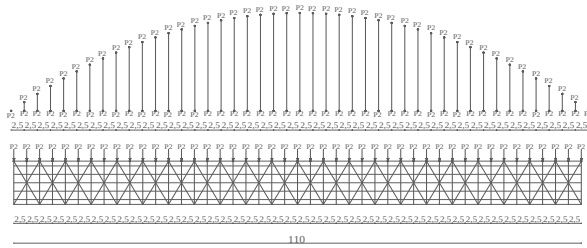
Gambar 10. Skema pembebanan angin pada kabel
