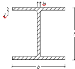
Gambar 11. . Penampang Baja WF
