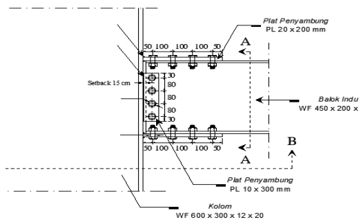
Gambar 6. Sambungan Induk - Kolom
