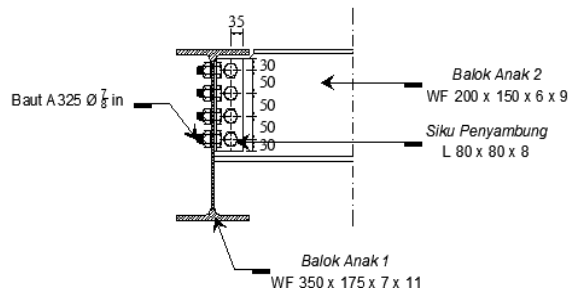
Gambar 5. Sambungan Anak 2 – Anak 1
