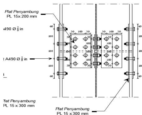
Gambar 7. Sambungan Kolom - Kolom
