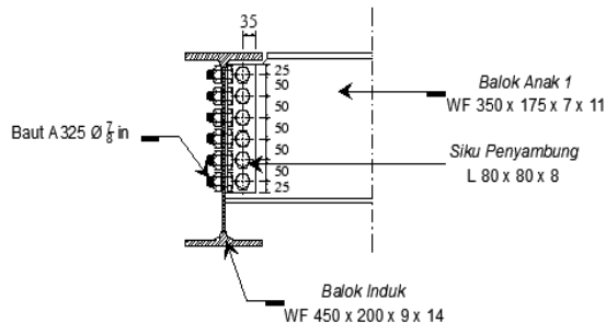
Gambar 4. Sambungan Anak 1 – Induk Kondisi 2
