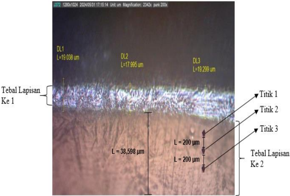
Gambar 4. Struktur mikro laju alir 60 cm 3 /min
