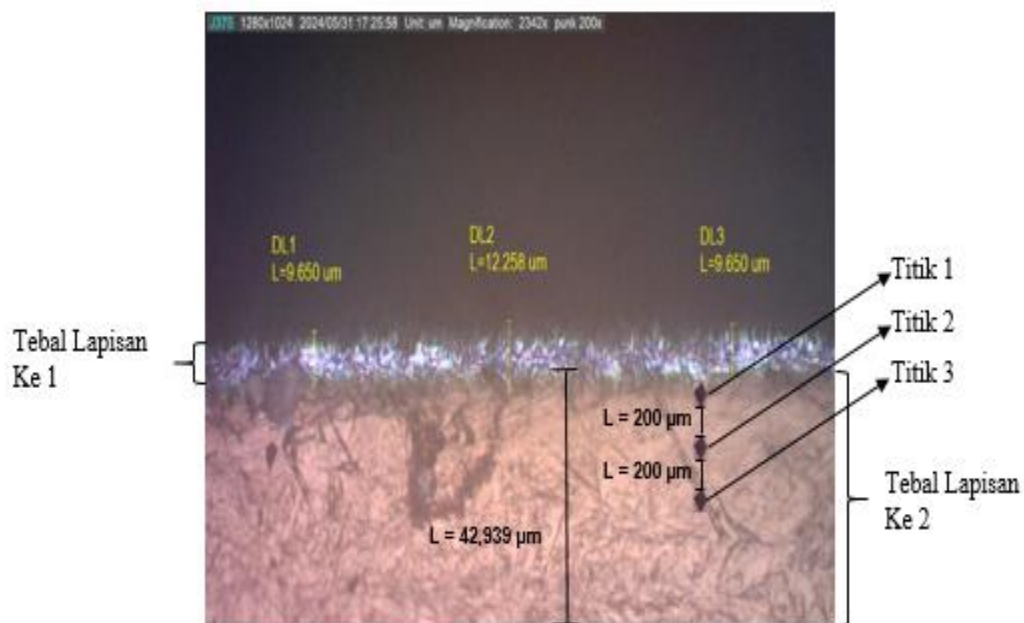
Gambar 2. Struktur Mikro Laju Aliran 20 cm 3 /min
