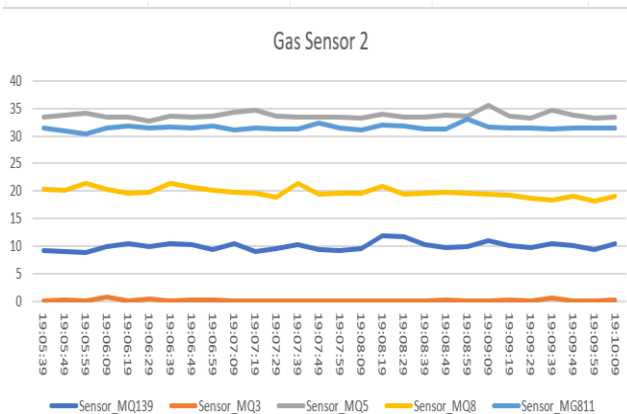
Gambar 46. Grafik Gas Sensor 2
