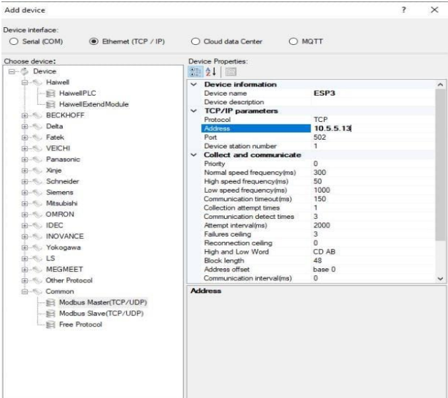
Gambar 27. Konfigurasi ESP 3
