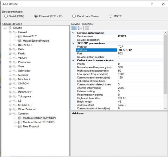
Gambar 26. Konfigurasi ESP 2
