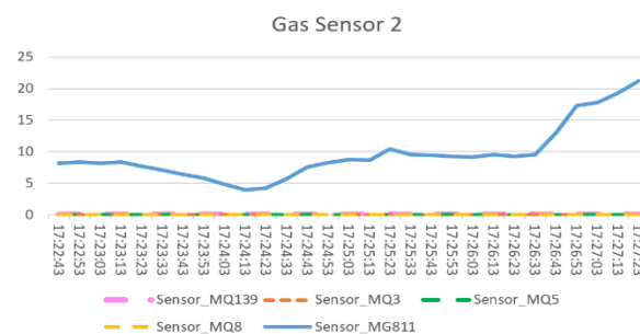
Gambar 40. Grafik Gas Sensor 2
