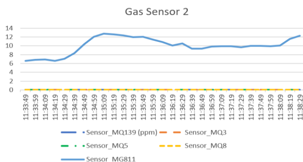
Gambar 37. Grafik Gas Sensor 2
