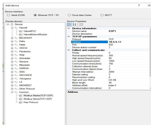
Gambar 25. Konfigurasi ESP 1
