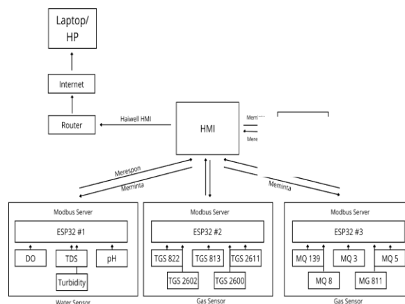
Gambar 16. Rancangan Keseluruhan Sistem
